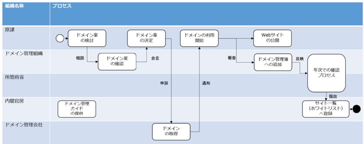
図 1. go ドメイン取得時の確認プロセス
